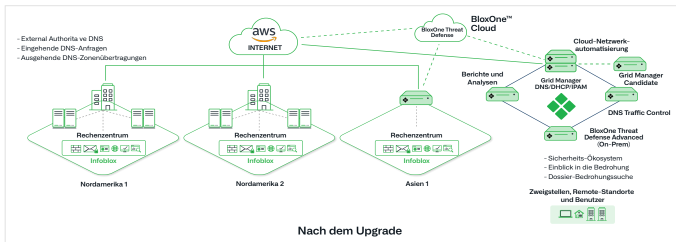
Abbildung 2: Architektur nach dem Upgrade mit modernisiertem DDI, einschließlich Reporting und BloxOne Threat Defense
