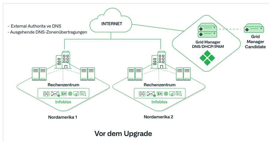
Abbildung 1: Netzwerkarchitektur vor der Modernisierung mit Infoblox
